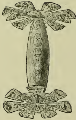
SODIUM.
